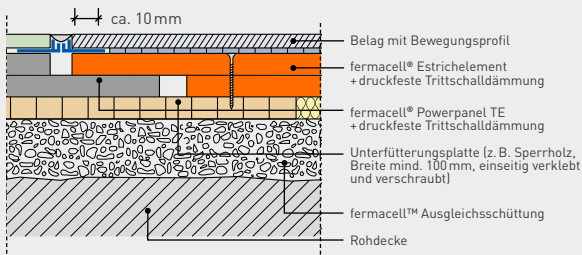
Bewegungsfuge auf fermacell™ Ausgleichsschüttung mit fermacell® Estrichelement oder Powerpanel TE Estrichelement
